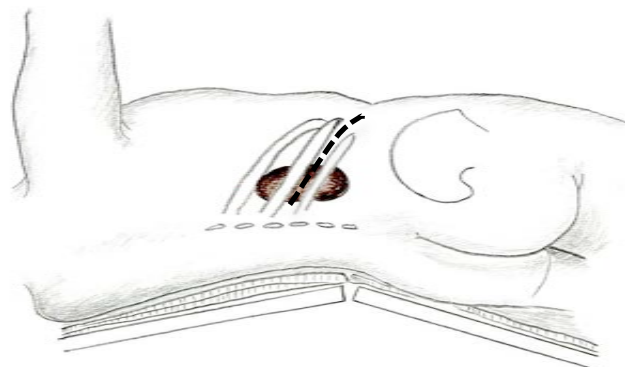
Klassische, offene Lebendspender-Nierenentnahme über Flankenschnitt
