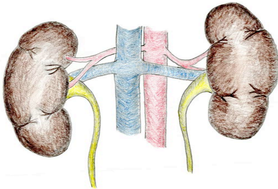
Anatomie der Nieren: Arterien , Venen , Harnleiter
