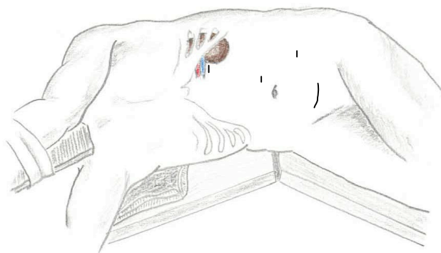
Minimalinvasive, laparoskopische Lebendspender-Nierenentnahme
