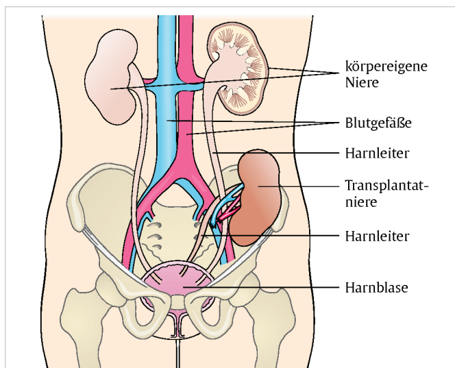
Abb.: Zustand nach der Nierentransplantation
